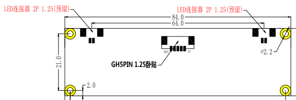
bot view
