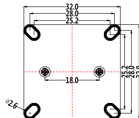
bot view
